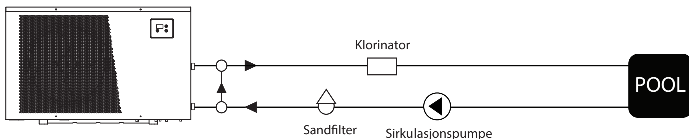
Prinsippkisse for installasjon av Q-serien
