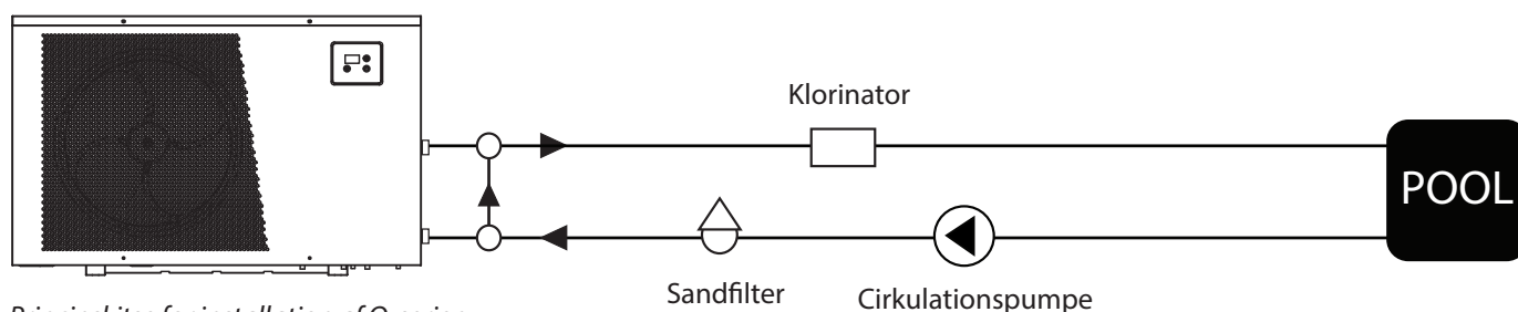
Principskitse for installation af Q-serien
